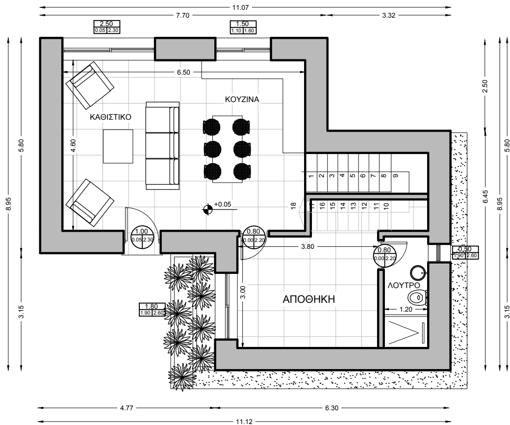
ΚΑΤΟΨΗ ΙΣΟΓΕΙΟΥ
