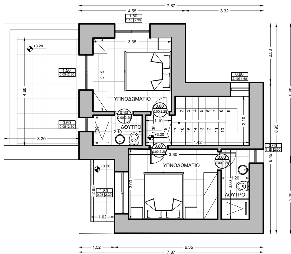
ΚΑΤΟΨΗ ΟΡΟΦΟΥ
