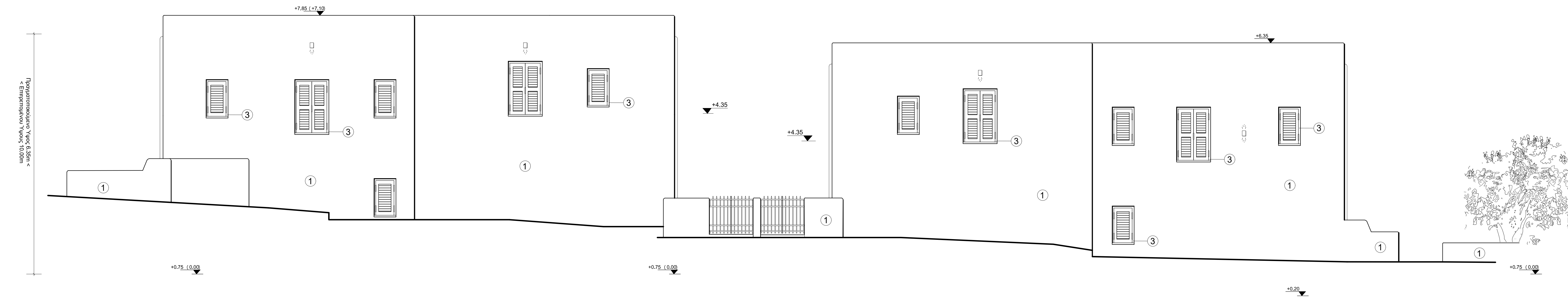
ΝΟΤΙΟΔΥΤΙΚΗ ΟΨΗ
